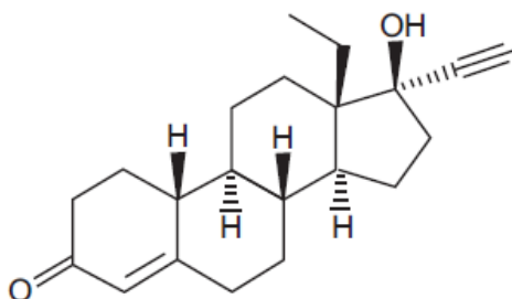
Norgestrel C 21 H 28 O 2 M.W. 312.5
